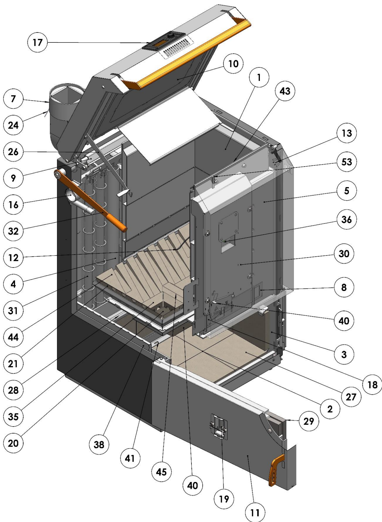
Schéma kotle – čelní pohled
