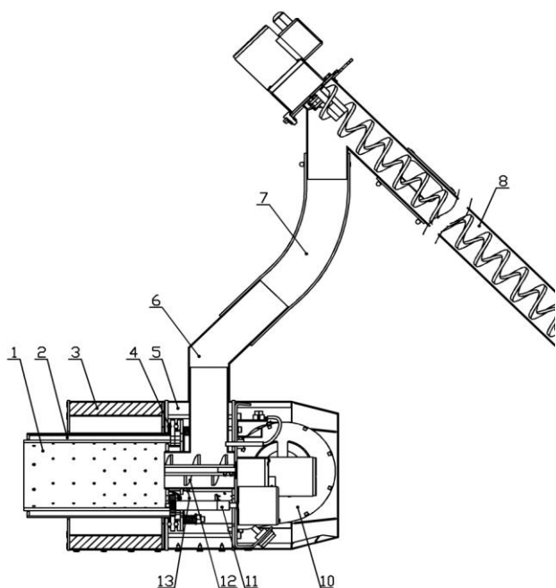
Schéma hořáku
