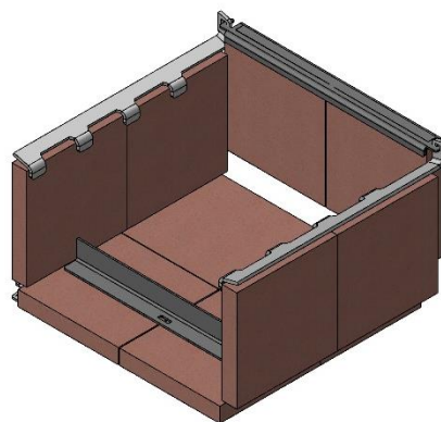
Spodní spalovací prostor - demonťovaná záslepka
