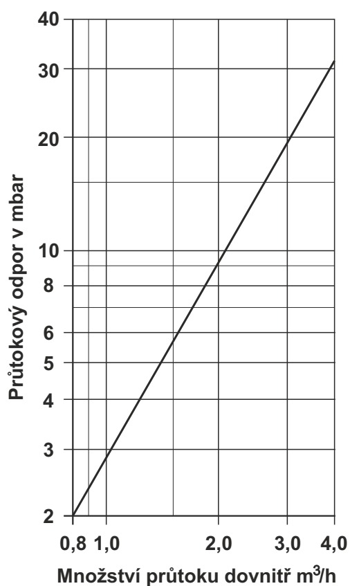
Obrázek 1. Průtokový odpor
