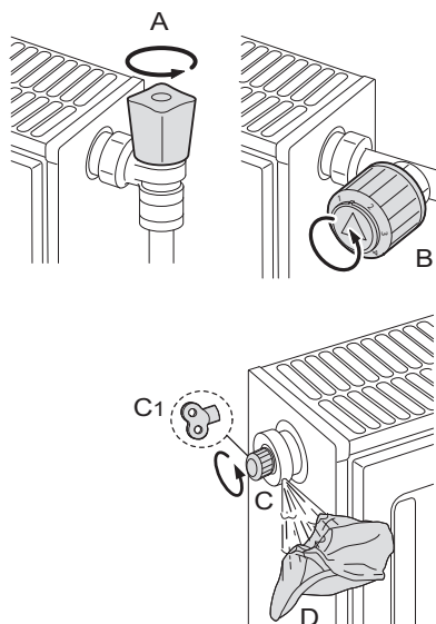
Obr.6 Čištění soustavy
