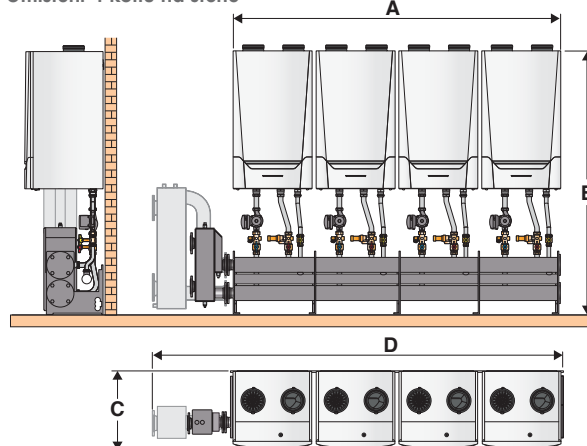
Umístění 4 kotlů na stěně
