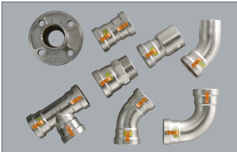
Obr. 1: Lisovací spojky Sanpress Inox G XL
