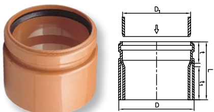
Přechodový kus KG PVC/kamenina – KGUSM
