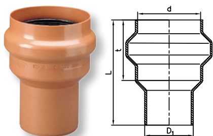
Přechodový kus kamenina/KG PVC – KGUS*
