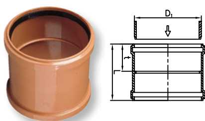
Spojka dvouhrdlá – KGMM
