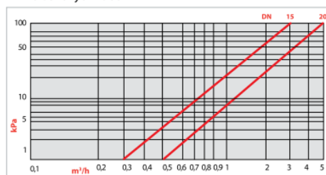
Křivka tlakových ztrát
