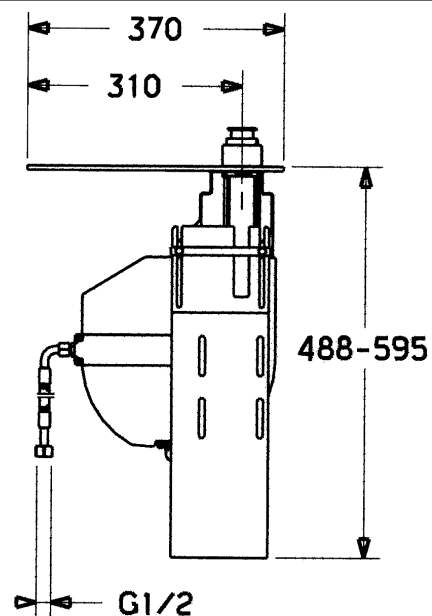
Výkres výrobku
