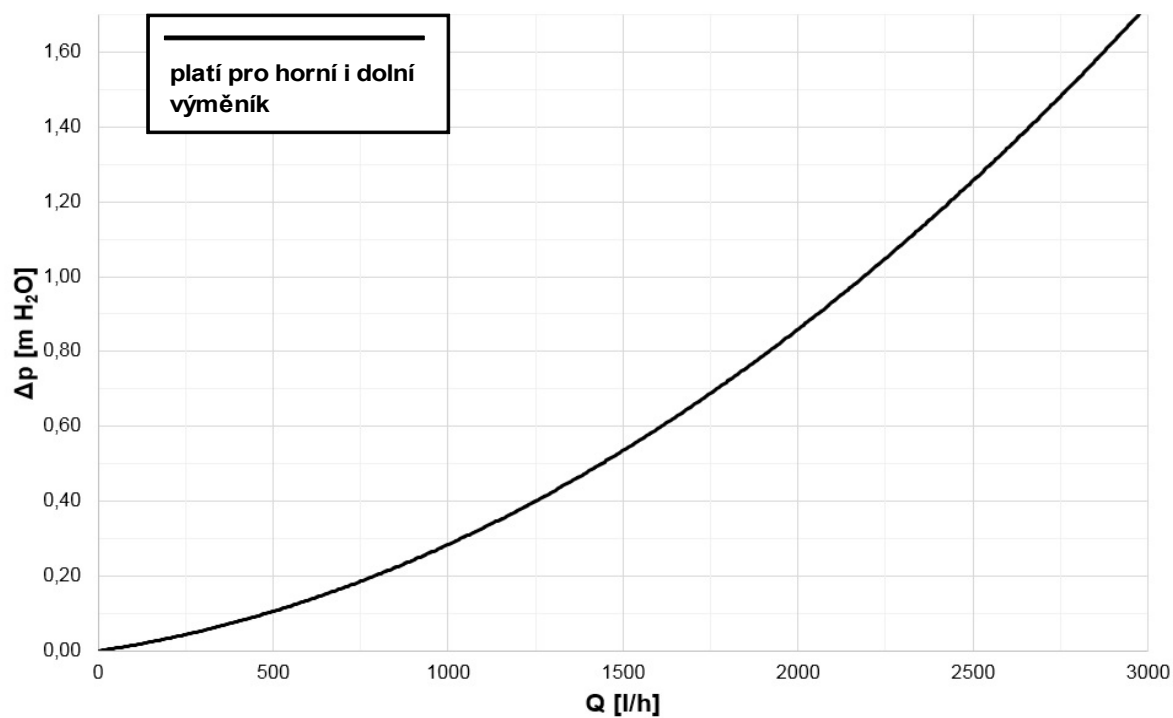
Graf tlakové ztráty výměníku
