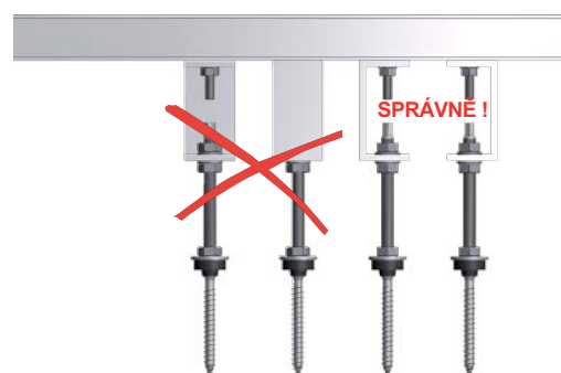
d) Šroub do střešní krytiny a jeho správné přichycení k „H“ profilu
