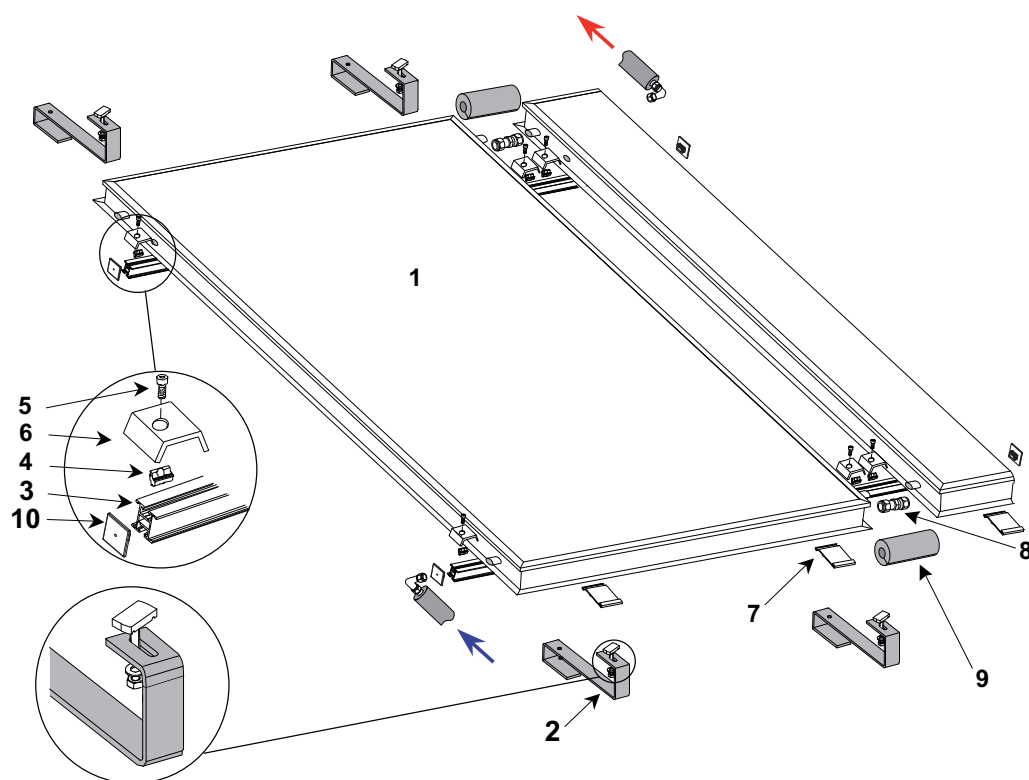
Obr. 1 Montáž kolektorů na šikmou střechu
