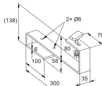
b) Střešní hák nerezový nebo z pozinkované oceli pro vlnité tašky
