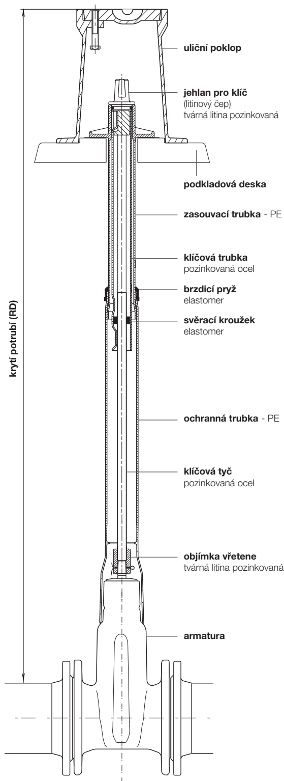
obrázek: teleskopická zemní souprava č. 9500A DN 80-200
