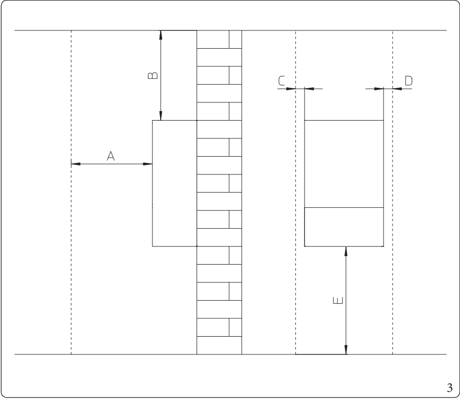
Vysvětlivky (Obr. 3): A - 450 mm B - 350 mm C - 30 mm D - 30 mm E - 350 mm
