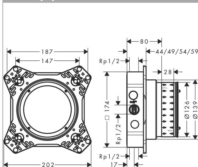
Kótovaný výkres
