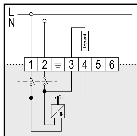
zapojení OCC2-1999H
