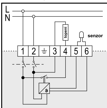
zapojení OCC2-1991-VS
