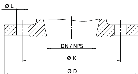
Obr. 5: Rozměry přírub
