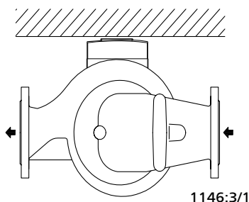
Obr. 8: Horizontální montáž (např. pod stropem)
