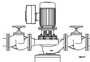
Obr. 11: Vertikální montáž / Upevnění s patkou čerpadla (příslušenství, je možné na vyžádání)
