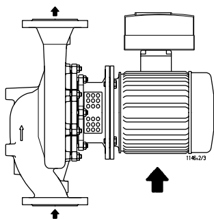
Obr. 6: Horizontální montáž, směr průtoku zdola nahoru
