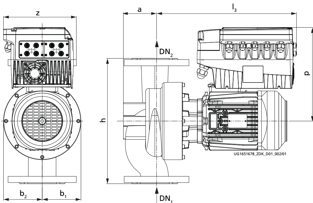
Obr. 3: Rozměry čerpacího agregátu s PumpDrive 2 Eco, s přírubovou přípojkou, konstrukční velikost < 032-032-100
