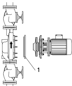
Obr. 9: Horizontální montáž pomocí zaslepovací příruby (1 = zaslepovací příruba, příslušenství)
