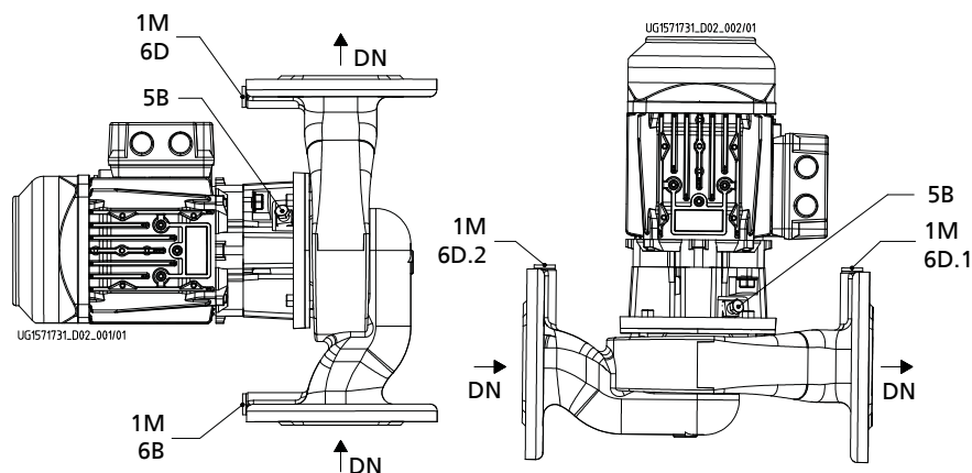
Obr. 4: Připojení
