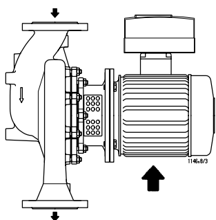
Obr. 7: Horizontální montáž, směr průtoku shora dolů
