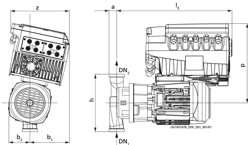
Obr. 2: Rozměry čerpacího agregátu s PumpDrive 2 Eco, se závitovou přípojkou, konstrukční velikost < 032-032-100
