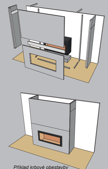
Příklad krbové obestavby celkově provedené z desek SKAMOTEC 225.
