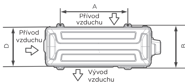
Pohled shora
