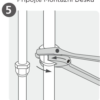
Připojte Potrubí
