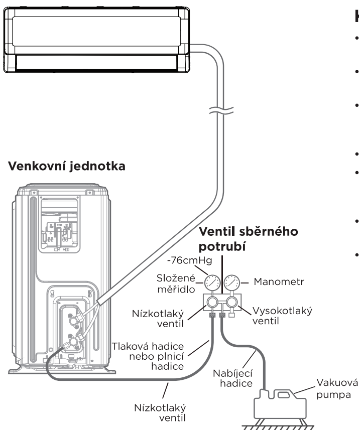
Vnitřní jednotka
