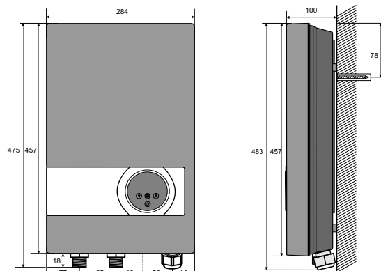
Okótovaný obrázek HAKL 3F-V
