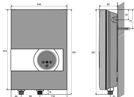
Okótovaný obrázek HAKL 3F-M
